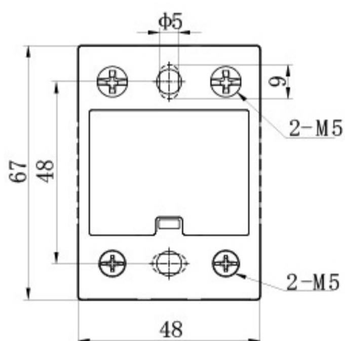
安装尺寸
